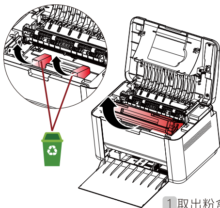
1 取出粉盒缓冲压块，取出粉盒
