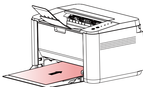
3 放入纸张
