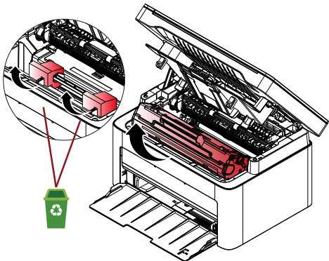
1 取出粉盒缓冲压块，取出粉盒
