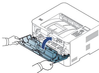
11. 合上前盖
